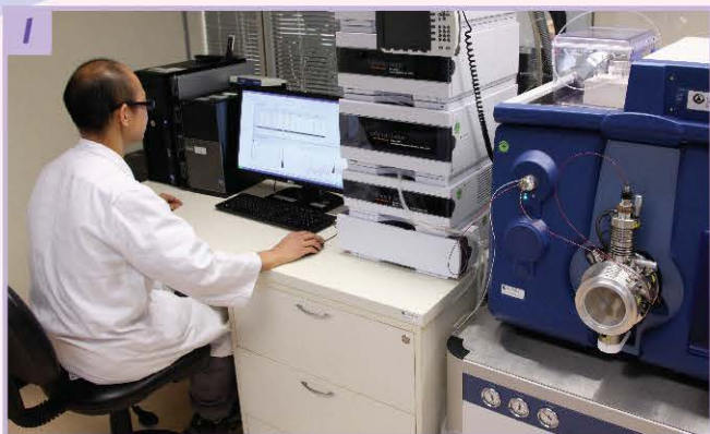
1 政府化驗所人員使用液相色譜/串聯質譜儀檢測食品中的天然毒素(如霉菌毒素)
